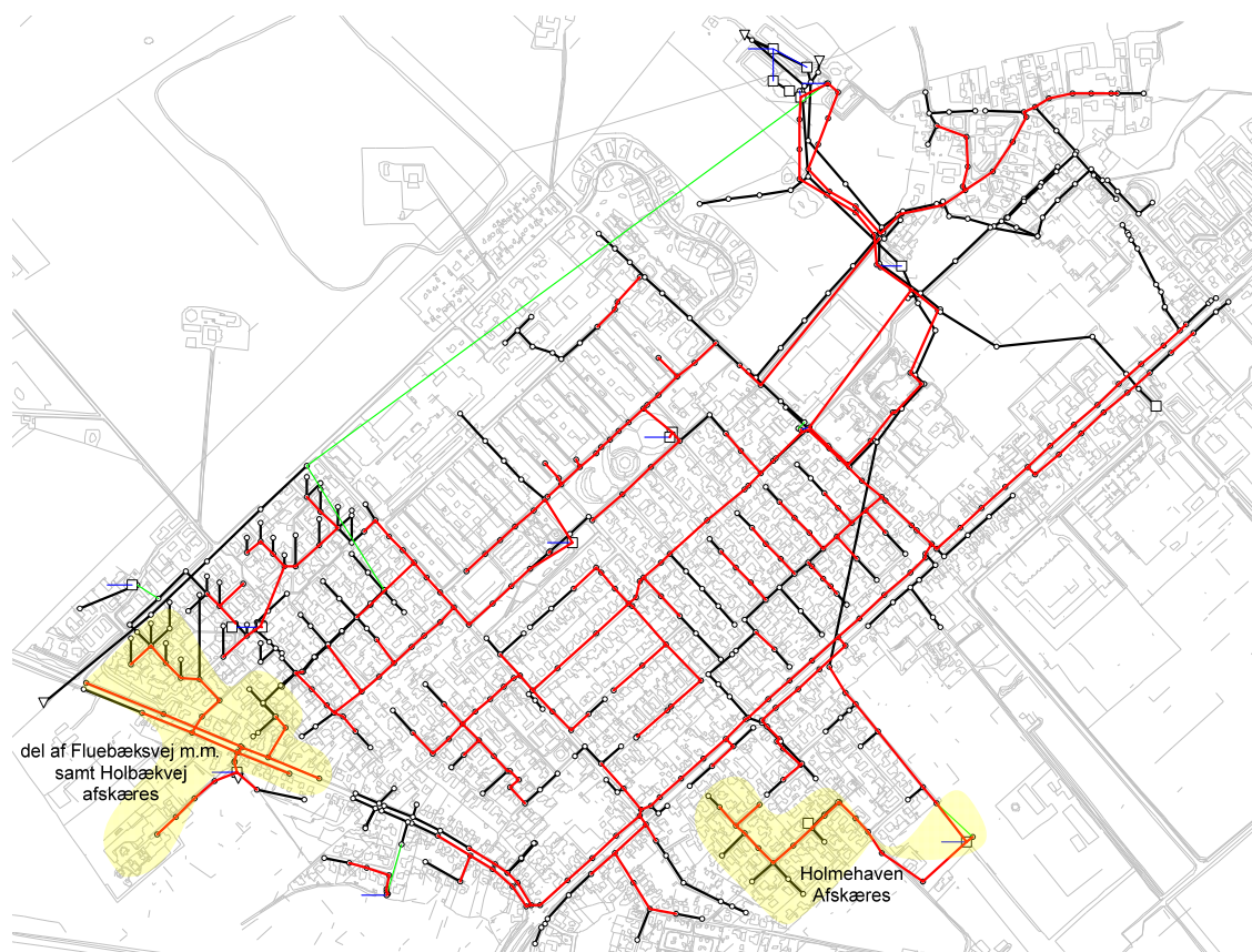
Figur 4. Behov for nye ledninger samt opdimensionering, såfremt eksisterende fællessystem bibeholdes.
