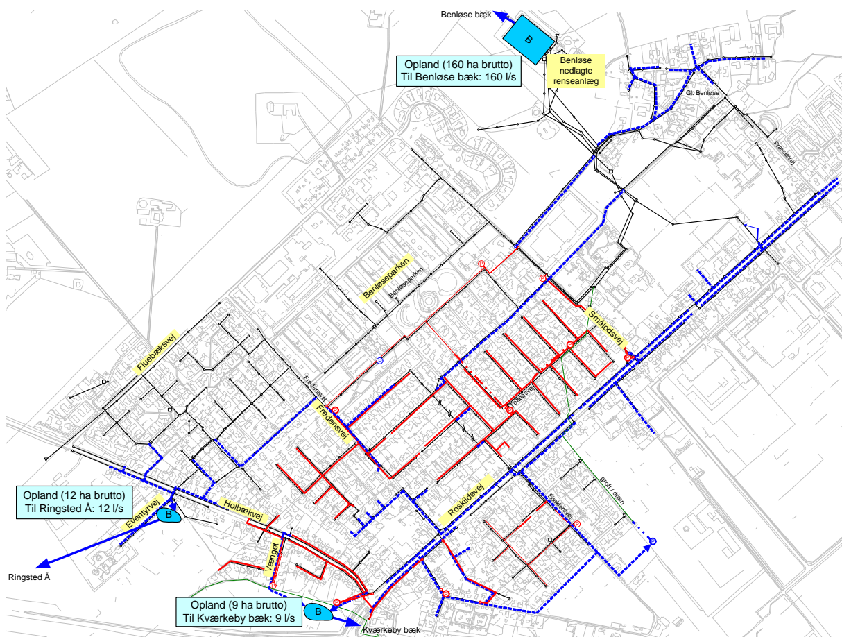
Figur 6. Forslag til kloakseparering af Benløse, med angivelse af forslag til bassiner med udløb til recipient. Opstuvningsbassiner er ikke vist. Anslået tilsluttet bruttoareal og forventet maks. udløbs-flow er vist i tekstboks. Der er kalkuleret med et afløbstal på 1 l/s/brutto-ha opland.
