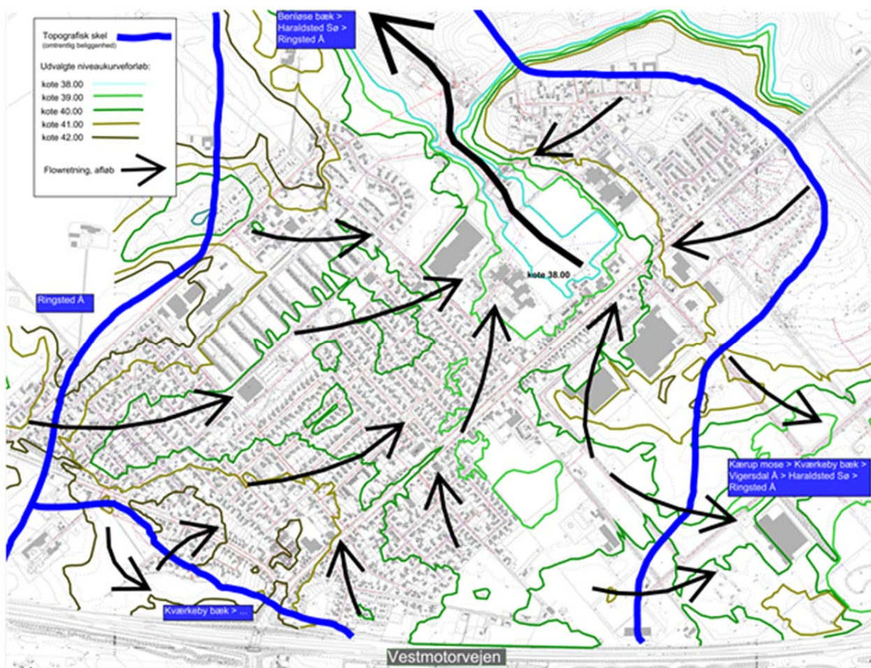
Figur 1 Oversigt over Benløses topografiske skel med angivelse af retning og recipient for regnvand/overfladevand. Udvalgte niveaukurver er trukket op.
